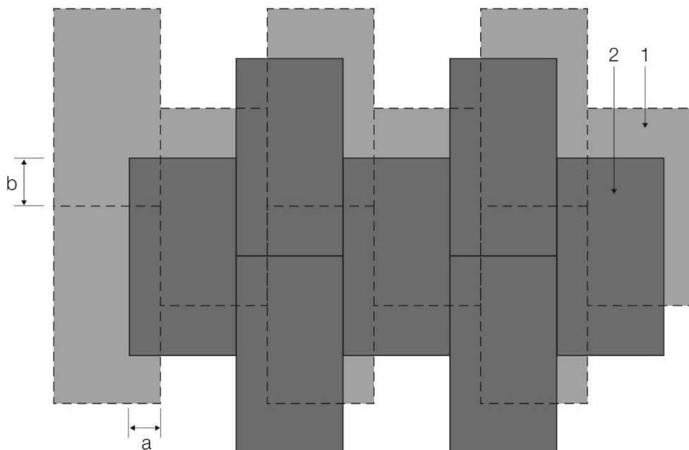
Figuur 14 - Aanbevolen legschema voor meerlaags isolatiesysteem op beton of hout ( a \geq 150 \text{ mm} – b \geq 150 \text{ mm} )
